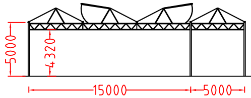
Doorsnede
