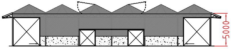
Aanzicht achtergevel
